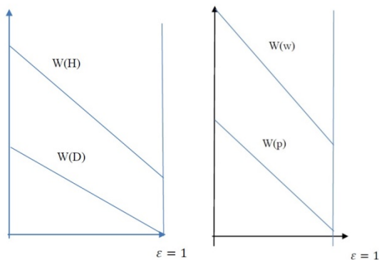
شکل ۱. نمودار تابع W
