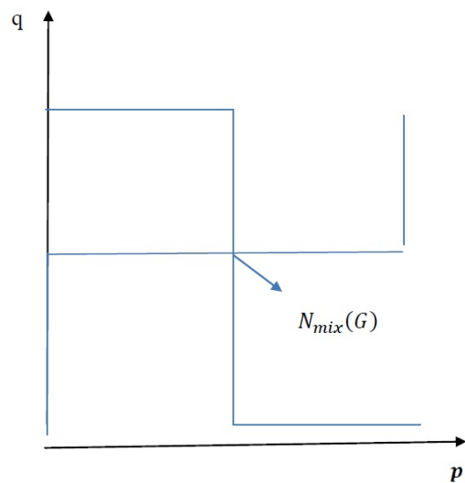
شکل ۲. تعادل نش مختلط
